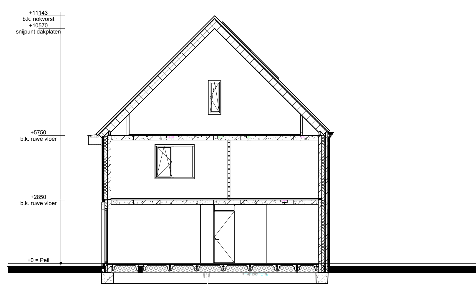
Doorsnede A3-A3
