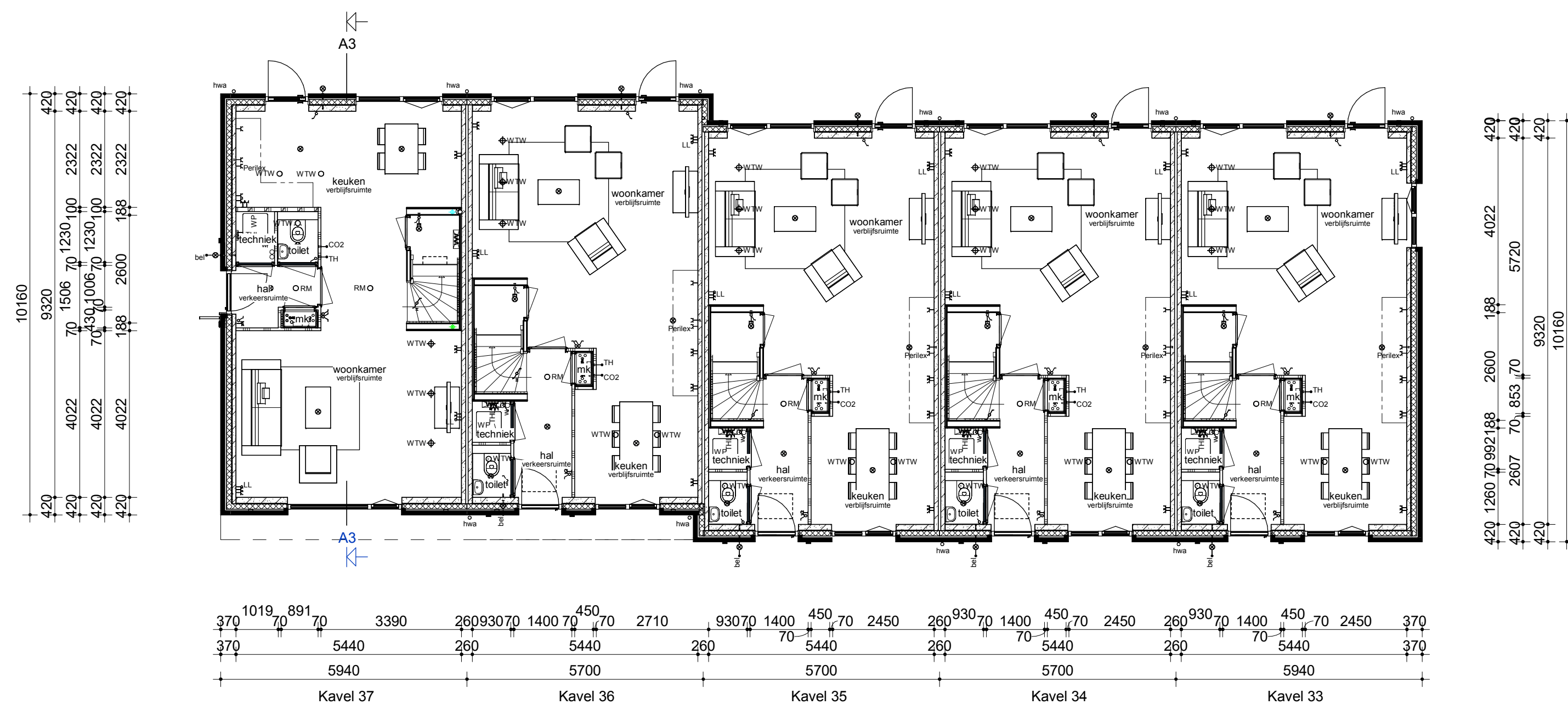
Begane grond
