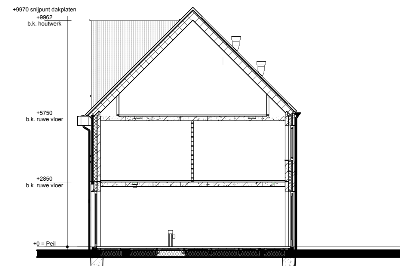
Doorsnede A1-A1
